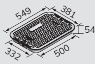
Regards de vanne rectangulaires 13" x 20"
