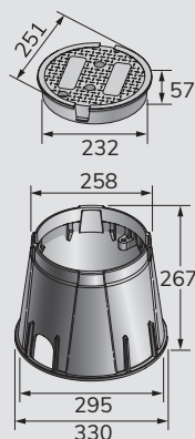
Regards de vanne métalliques 10"
