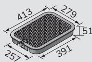
Regards de vanne rectangulaires 14" x 19"
